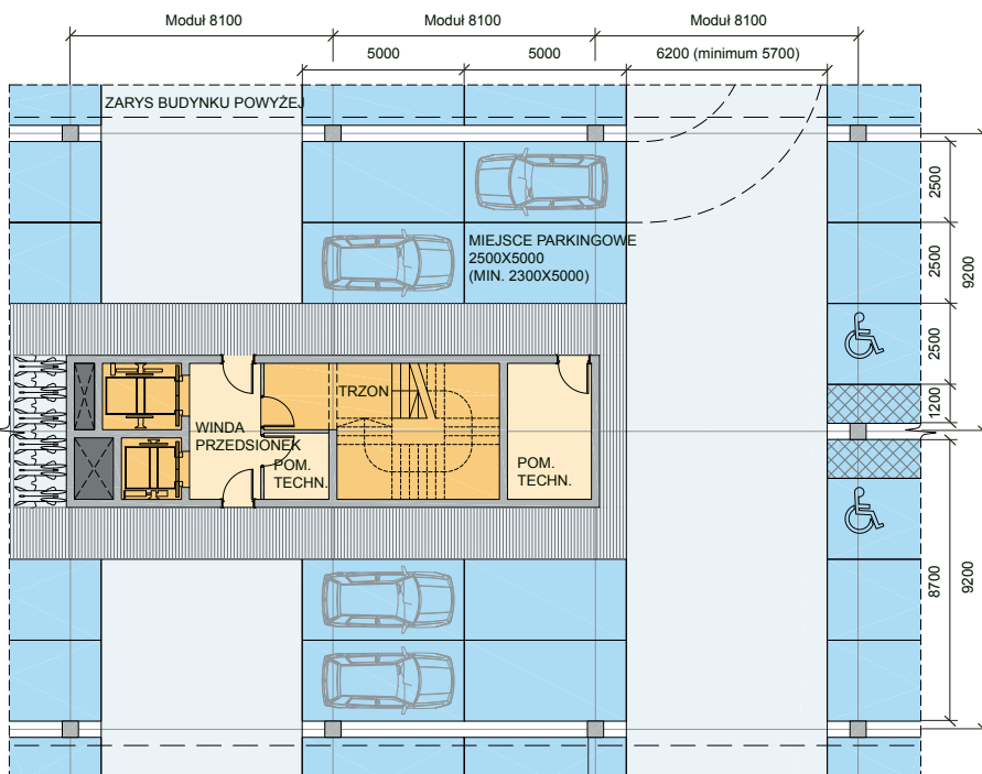
Siatka projektowa i konstrukcyjna – rzut parkingu podziemnego
